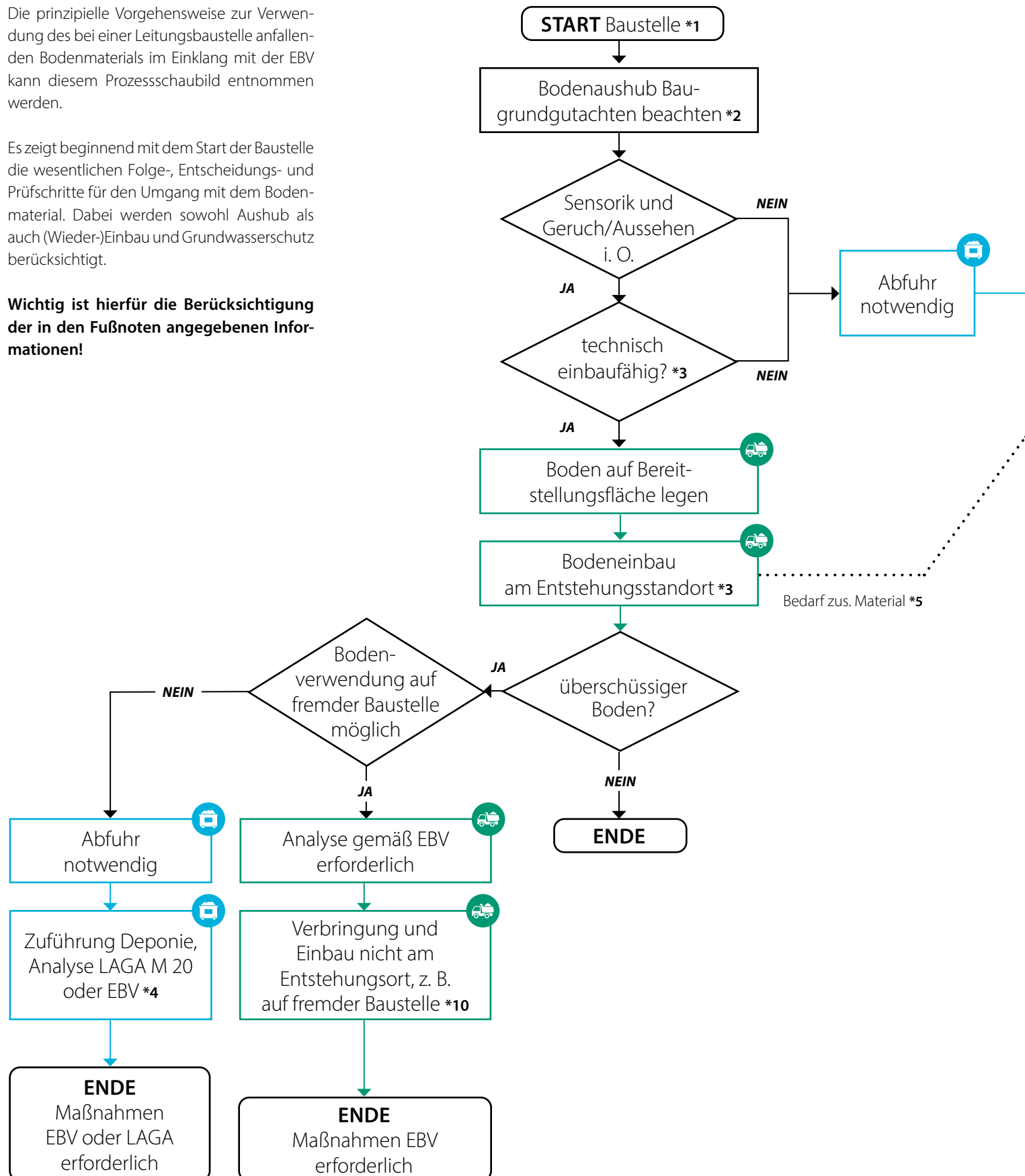
Abbildung 4: Prozessschaubild zur Verwendung von Bodenmaterial im Einklang mit der EBV
